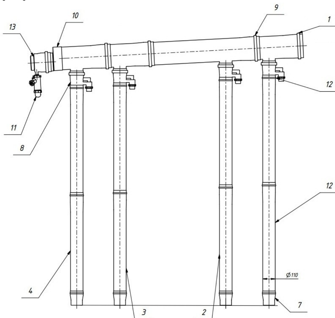
Рис. 2. Комплект каскадных дымоходов Тип 2
