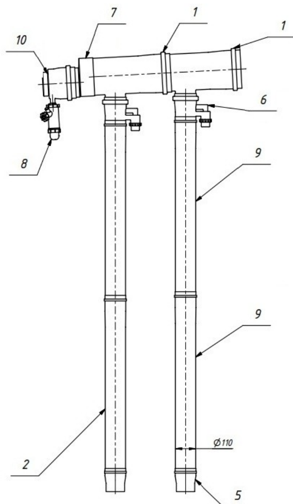
Рис. 3. Комплект каскадных дымоходов Тип 3
